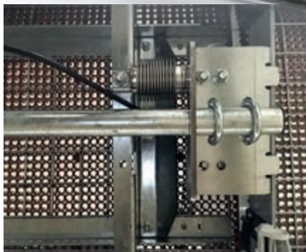
Тензометричен датчик
