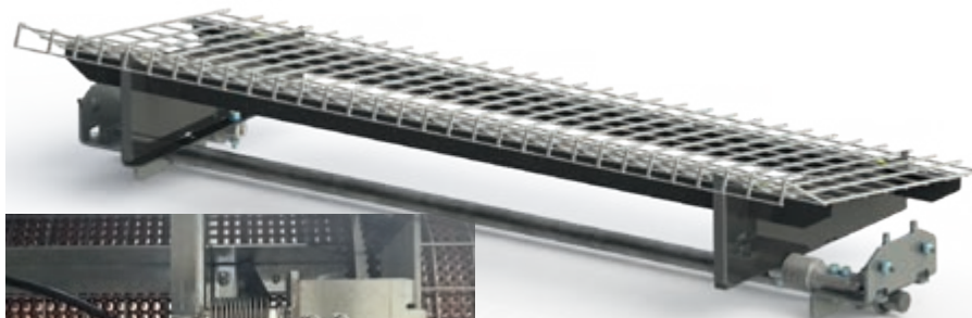
Монтиране на кантара Nesca 2 под пода на гнездото
