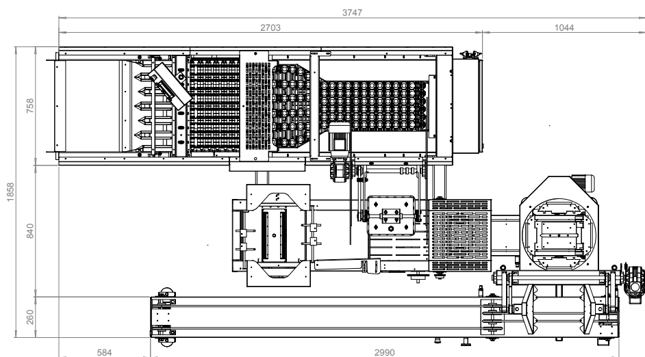
PrimePacker 100 con apilador de bandejas
