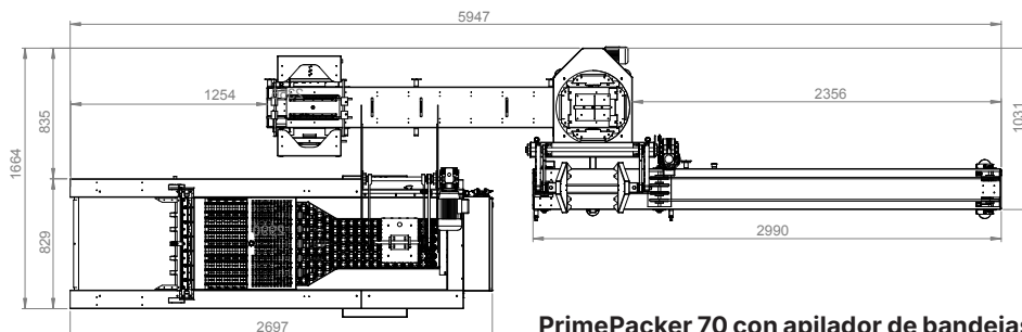
PrimePacker 70 con apilador de bandejas
