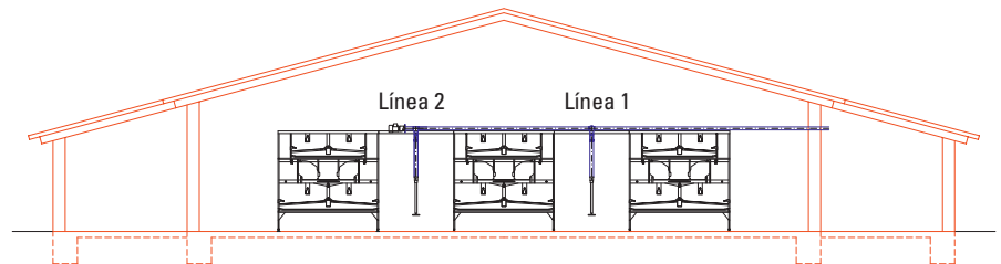
Sección transversal de la nave: PickPuck con llenado automático
