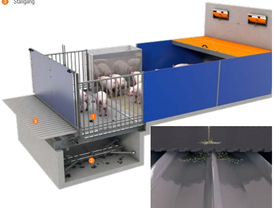
Querschnitt durch eine Bucht
