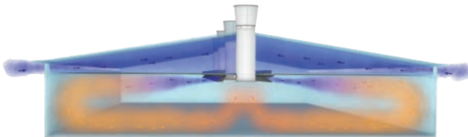
Der Einbau kann auch in Stallmitte erfolgen, wenn es dort am wärmsten ist
