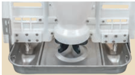
La unidad dosificadora no toca el fondo del comedero → buena higiene de pienso
