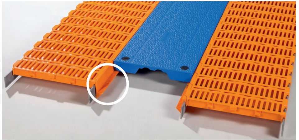
Ejemplo de montaje: integración fácil de una placa de calefacción mediante listones
