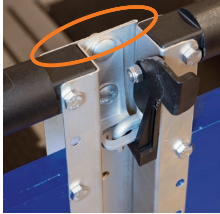
Soporte reforzado en la zona de la puerta
