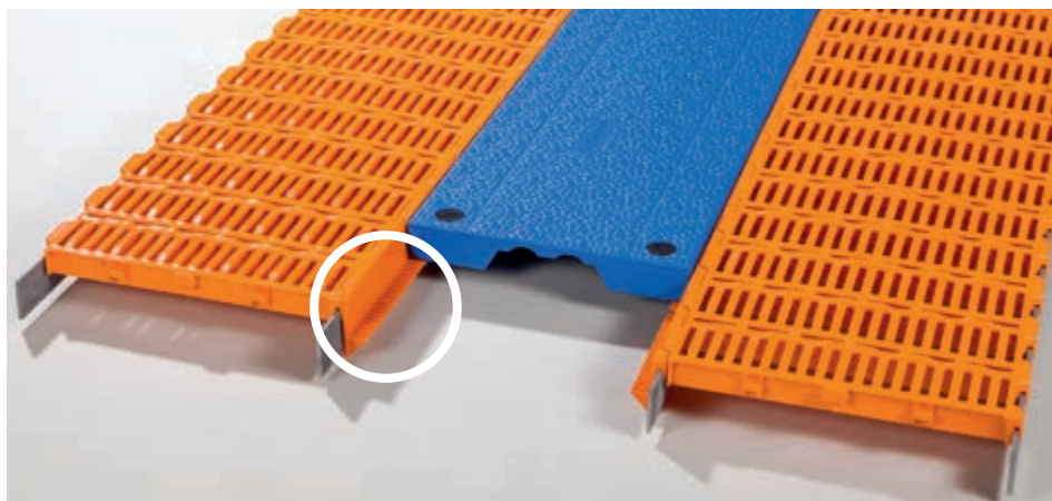
Primjer ugradnje: Jednostavna ugradnja grijaće ploče zahvaljujući nosačima za podupiranje
