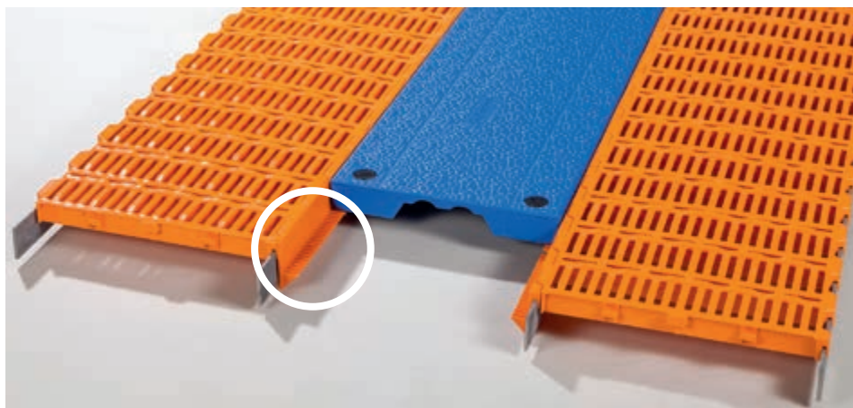
Przykład montażu: proste łączenie płyty grzewczej za pomocą listew
