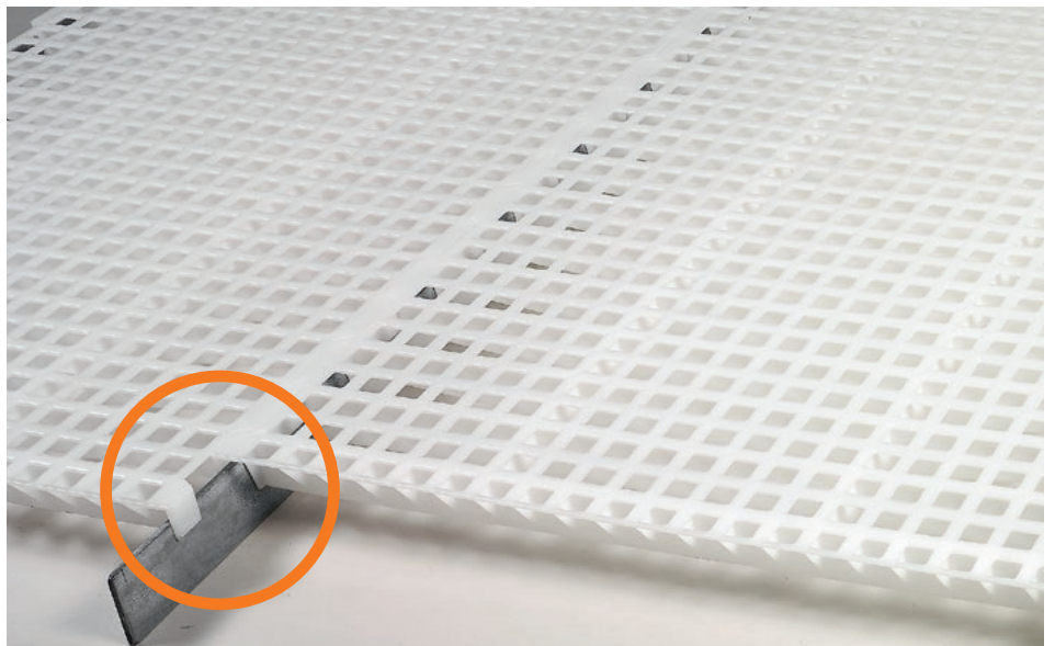
Les caillebotis se montent sur des fers plats standard de 60 x 5 mm. Ils présentent une portée maximum de 3 m.
